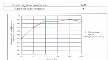
Рисунок 2 Диаграмма значений фактического коэффициента звукопоглощения \alpha_w
