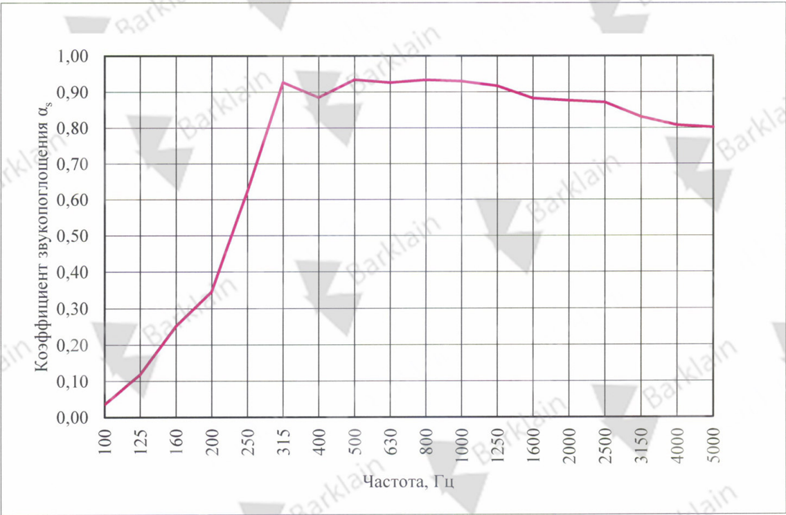
Рисунок 1 Диаграмма значений коэффициента звукопоглощения \alpha_s
